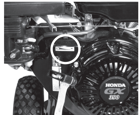
Figura 10 - Obturador
