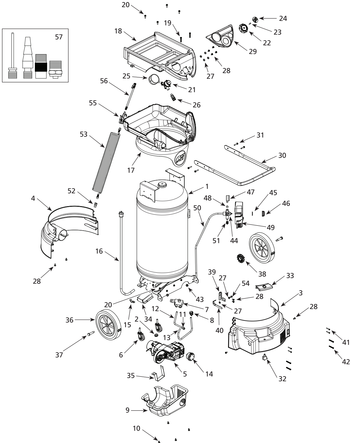
Figure 21 – Illustration des pièces de réparation pour l'ultime compresseur d'air de garage portable, modèle WL6701 et WL6703
