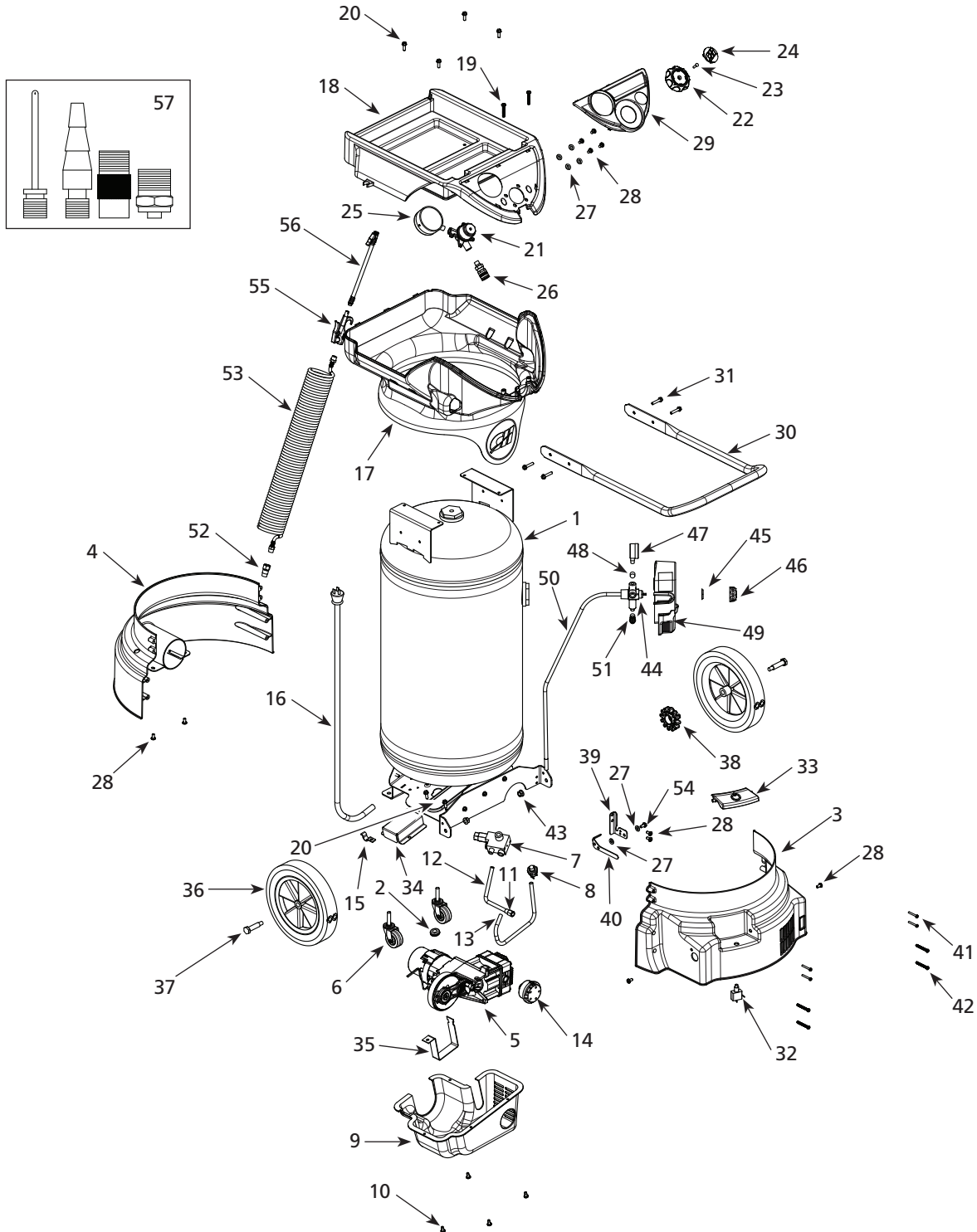
Figura 21 – Ilustración de las piezas de repuesto para el Máximo compresor de aire portátil para el garaje modelo WL6701 y WL6703
