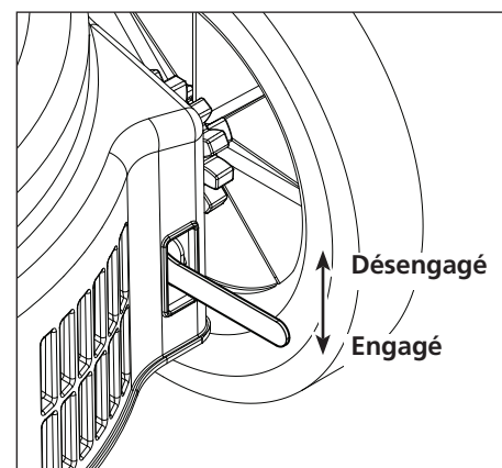
Figure 10 - Verrou de roue/frein à pied
