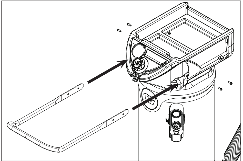
Figure 9 - Assemblage de poignée
