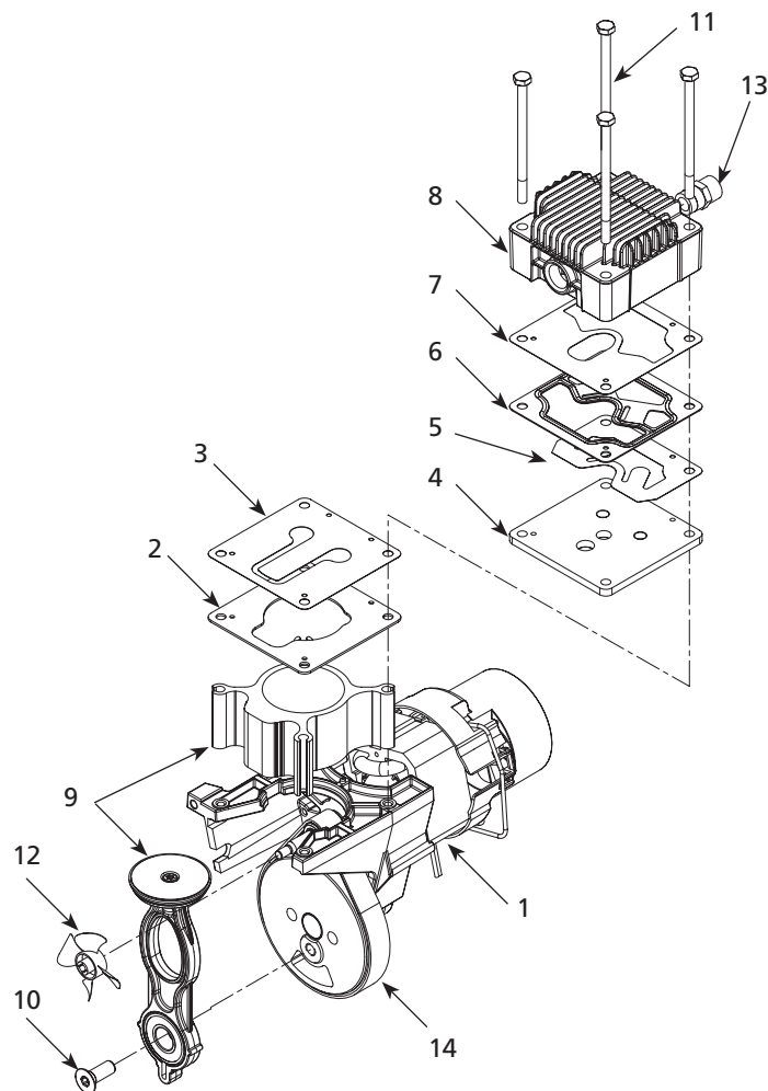
Figure 20 – Illustration des pièces de rechange de la pompe, modèle WL390100
