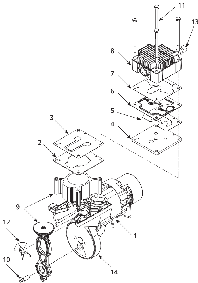
Figura 20 – Ilustración de Piezas de repuesto para bomba, modelo WL390100
