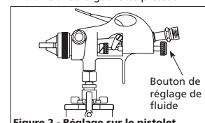
Figure 2 - Réglage sur le pistolet
