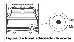
Figura 3 - Nivel adecuado de aceite
