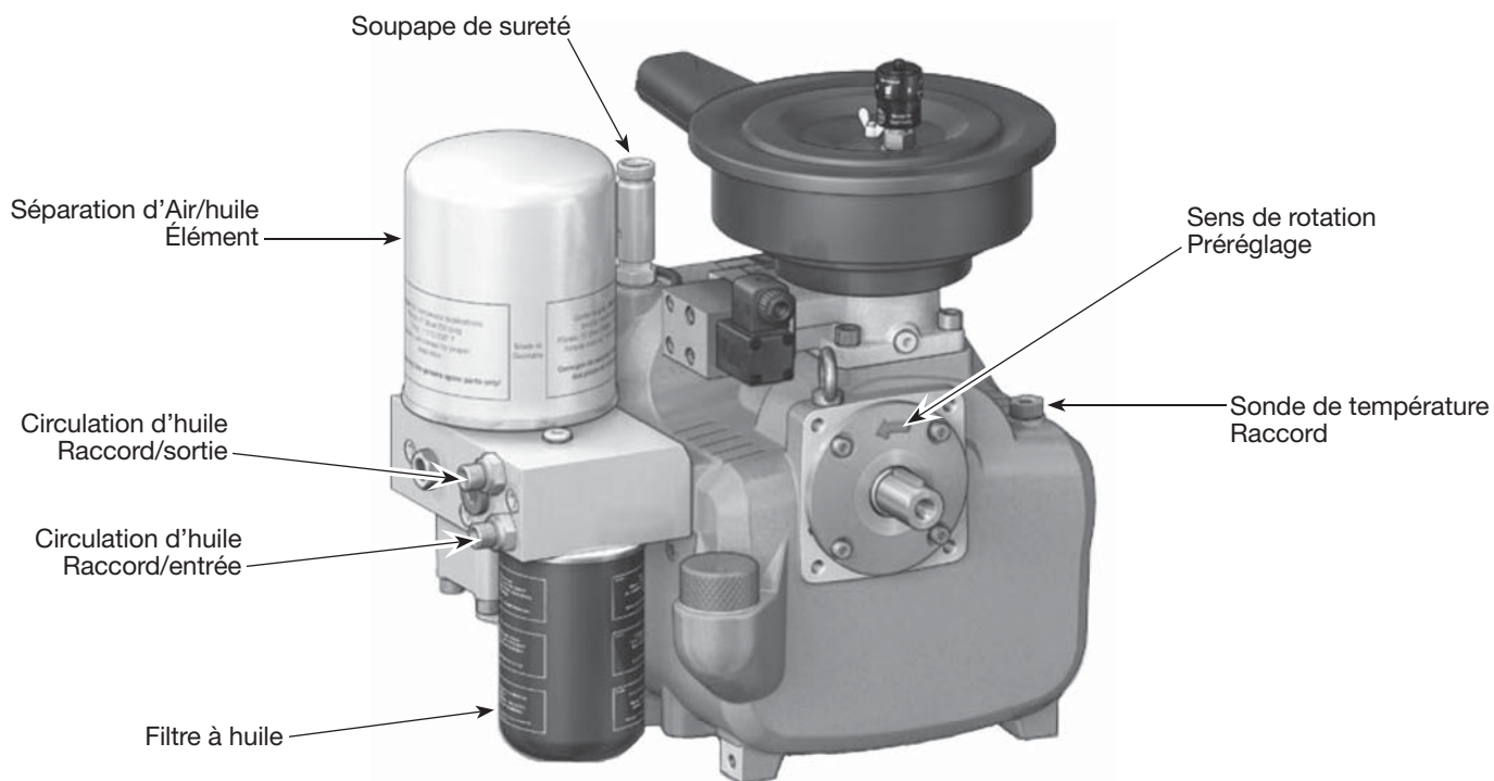
Figure 3 - Composants de l'extrémité air
