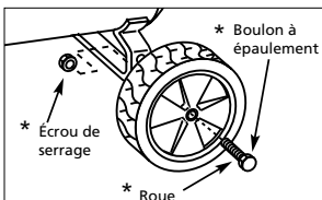
Figure 2 - Montage De Roues
