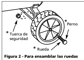
Figura 2 - Para ensamblar las ruedas
