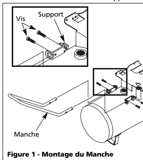
Figure 1 - Montage du Manche
