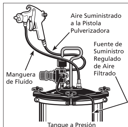
Figura 4 - Conexión del Tanque a Presión
