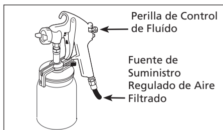
Figura 2 - Conexión del Sistema de Sifón
