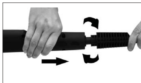
Figura 12 - Conecte la lanza a la pistola.
