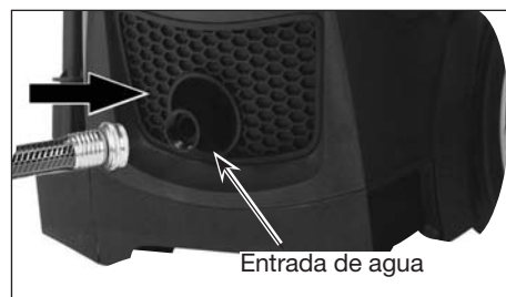
Figura 14 - Conecte la manguera de jardín a la unidad (modelos PW1625 y PW1835)
