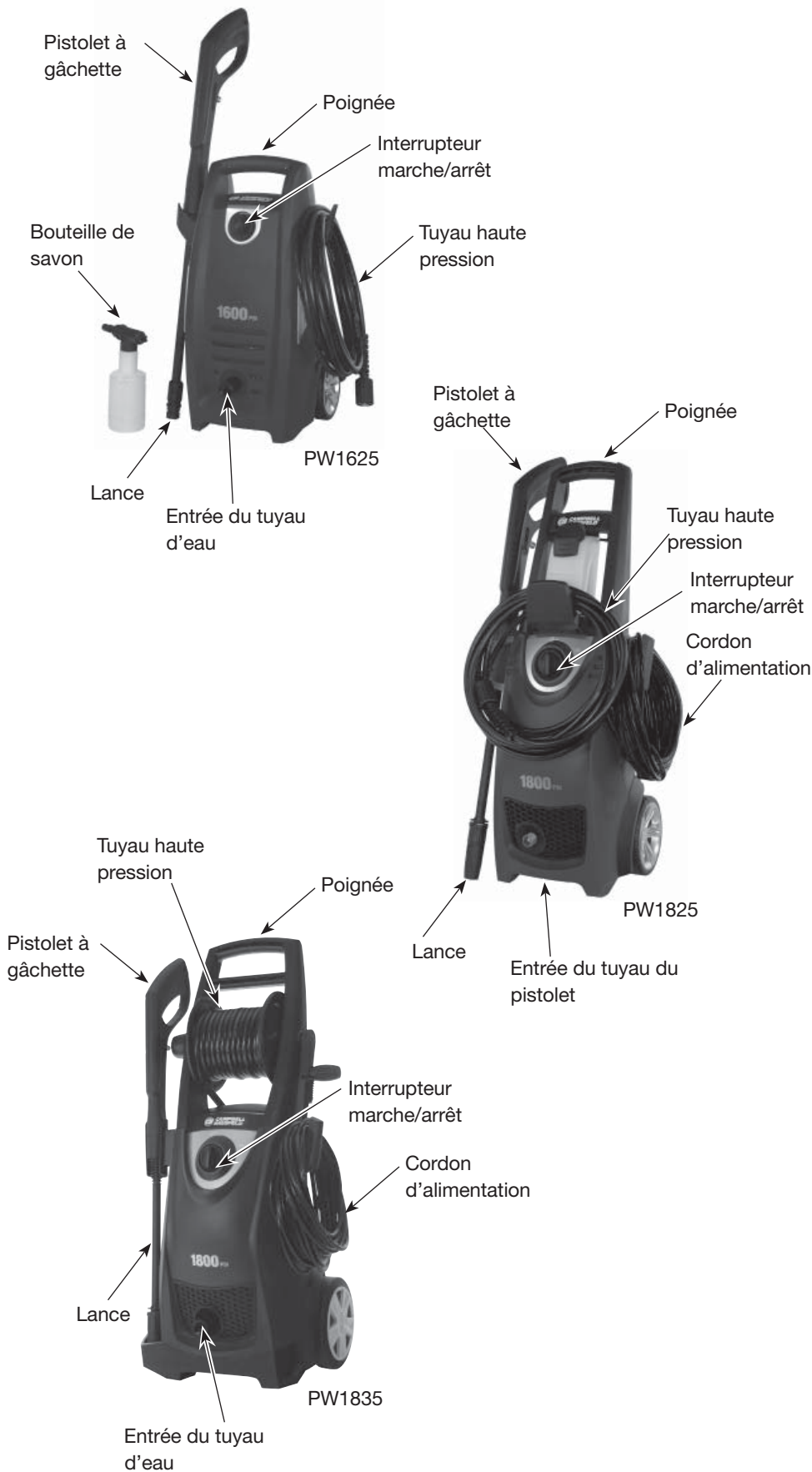
Figure 6 - Composants de laveuse à pression
