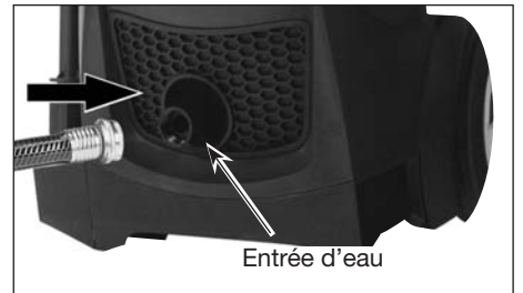
Figure 14 - Attachez le tuyau d'arrosage à l'unité (modèles PW1625 et PW1835)
