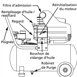
Figure 6 - Identification du modèle
