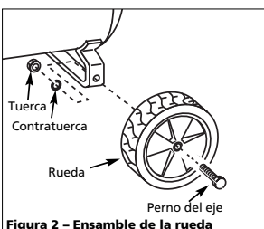
Figura 2 – Ensamble de la rueda
