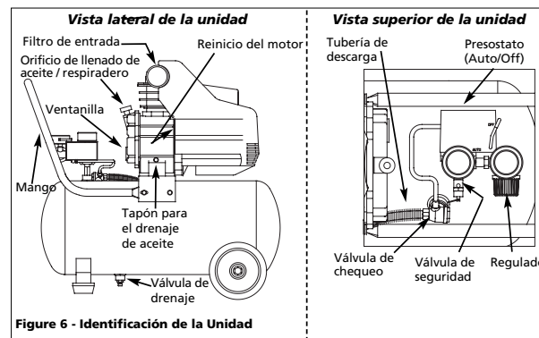
Figure 6 - Identificación de la Unidad
