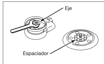
Figura 2 - Montaje de la almohadilla para lijar
