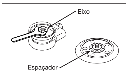
Figura 2 - Conjunto do bloco da lixa
