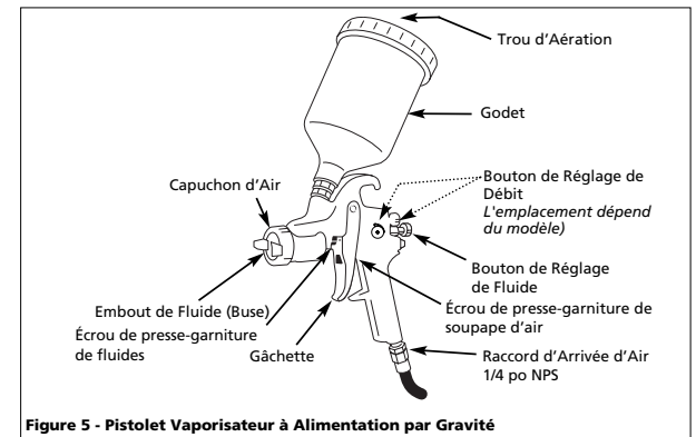
Figure 5 - Pistolet Vaporisateur à Alimentation par Gravité
