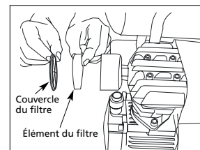
Figure 6 - Entretien du filtre d'aspiration
