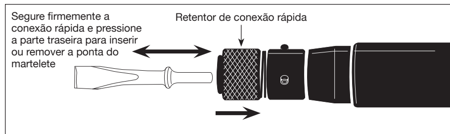
Figura 3 - Operação do retentor de conexão rápida
