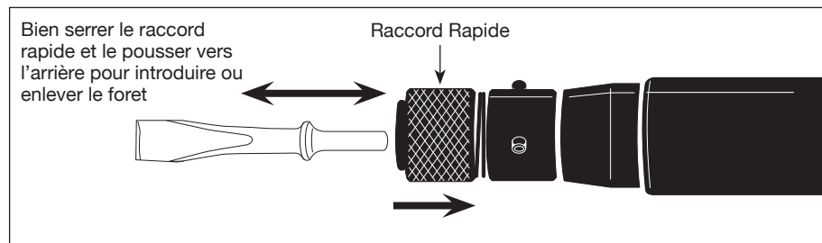
Figure 3 - Fonctionnement du Raccord Rapide
