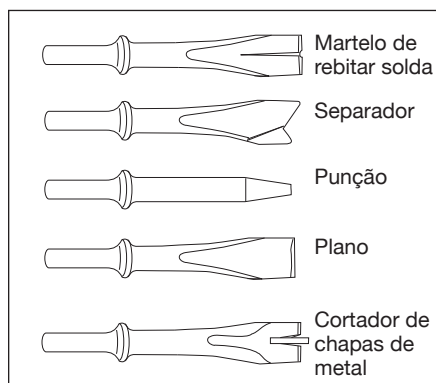
Figura 5 - Pontas de martelete
