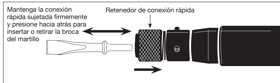
Figura 2 - Funcionamiento del Retenedor de Conexión Rápida
