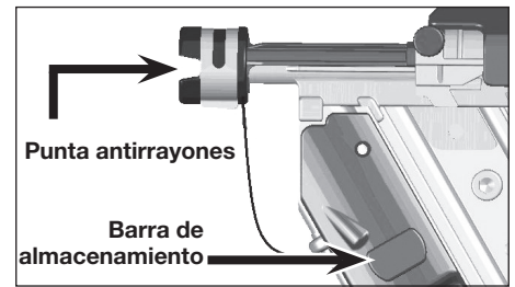
Figura 15 - Punta antirrayones
