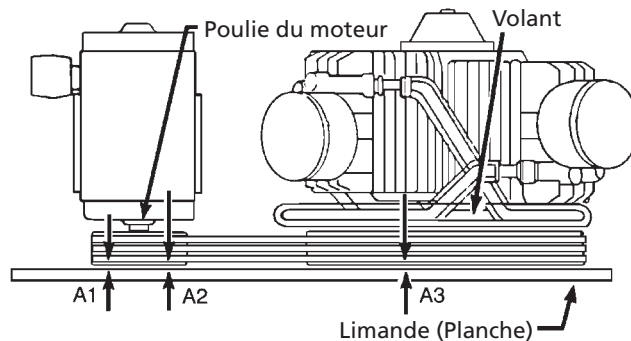
Figure 9 - Vue de dessus
