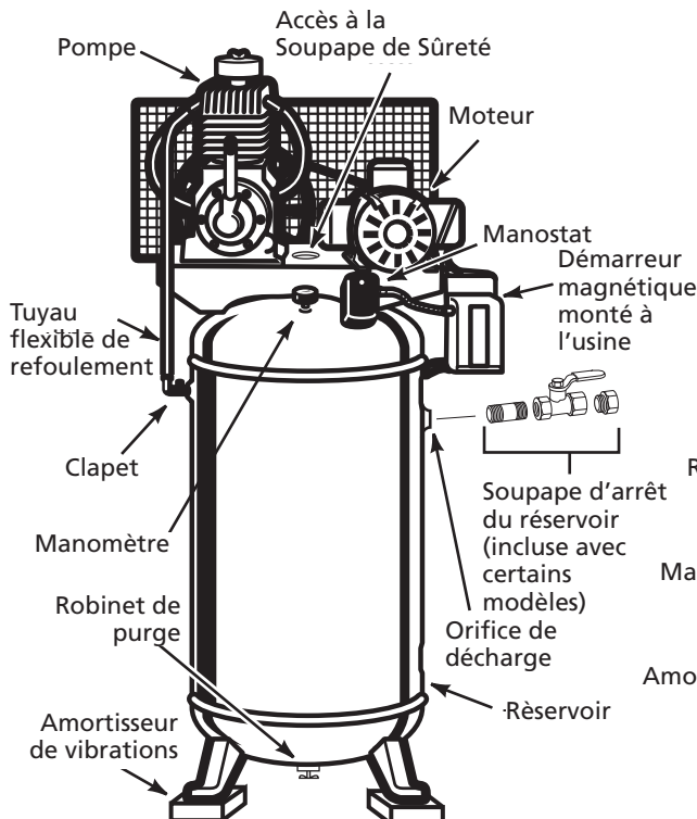
Figure 1 - Identification du Modèle Vertical
