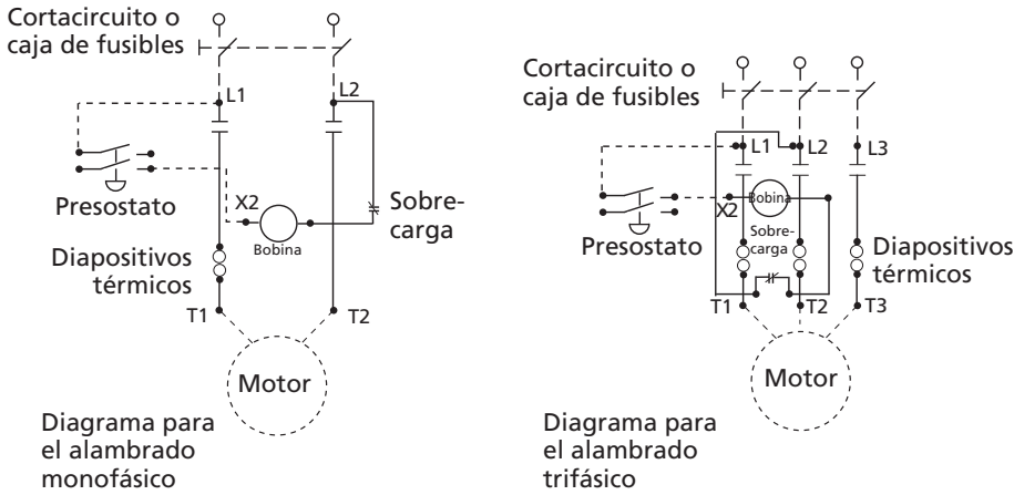
Figura 4 - Para los Motores con nomenclatura 184T, 215T, 254T ó 284T. Vea la placa del motor
