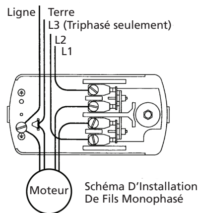
Figure 3 - Pour Les Moteurs De Taille R56HZ, Y56Y ou L143T. Se Référer À La Plaque Indicatrice Sur Le Moteur
