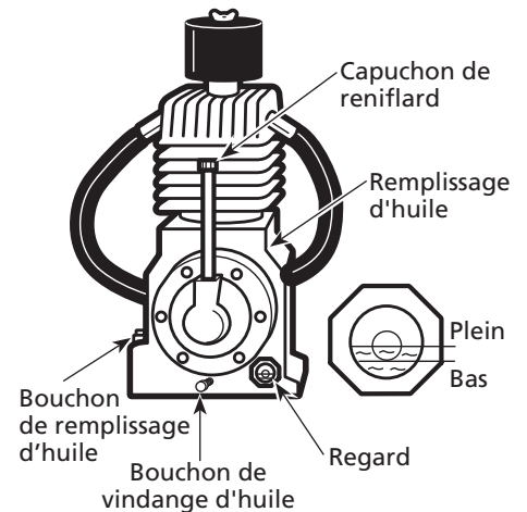
Figure 5 - Schémas De Remplissage D'Huile
