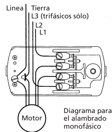
Figura 3 - Para los Motores con nomenclatura R56HZ, Y56Y ó L143T. Vea la placa del motor
