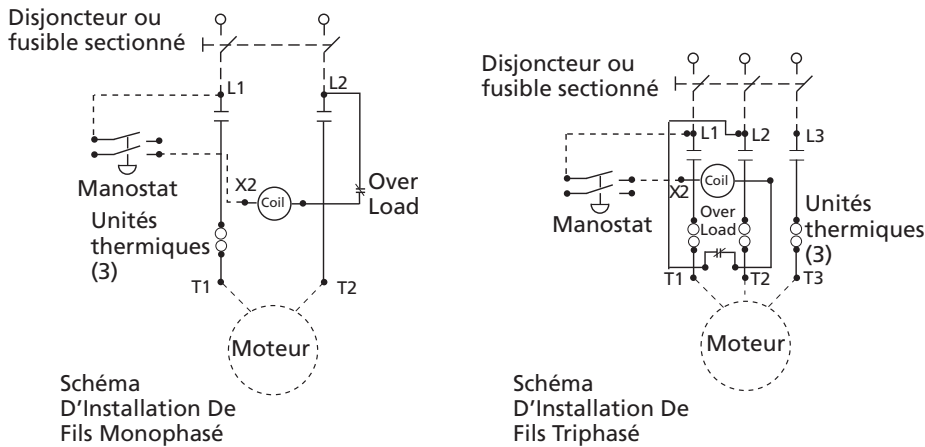
Figure 4 - Pour Les Moteurs De Taille 184T, 215T, 254T ou 284T. Se Référez À La Plaque Indicatrice Sur Le Moteur
