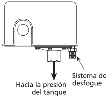
Figura 7 - Presostato
