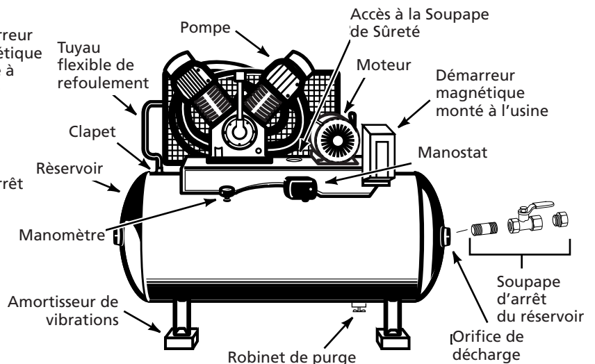
Figure 2 - Identification du Modèle Horizontal
