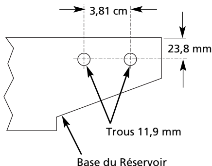
Figure 2 - Troux Percés
