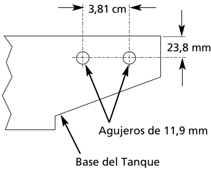
Figura 2 - Agujeros Perforados
