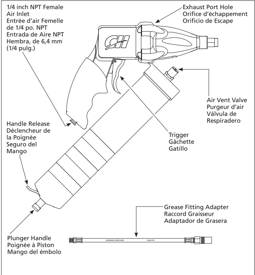
Figure 1 - Air Grease Gun Features Figure 1 - Caractéristiques du Pistolet Graisseur Pneumatique Figura 1 - Características de la Pistola Lubricadora Neumática
