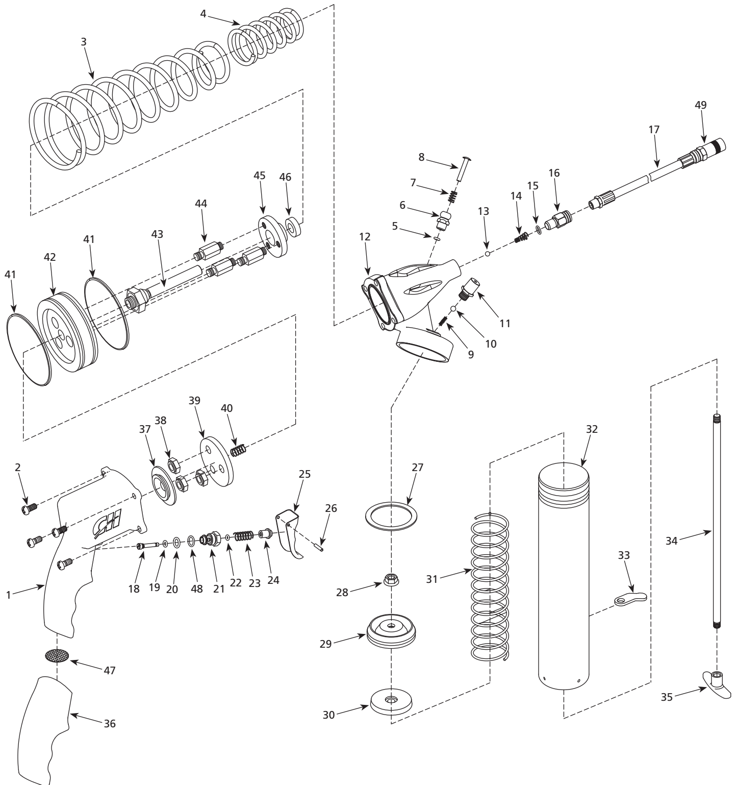
Figure 1 - Ilustración de los Repuestos
