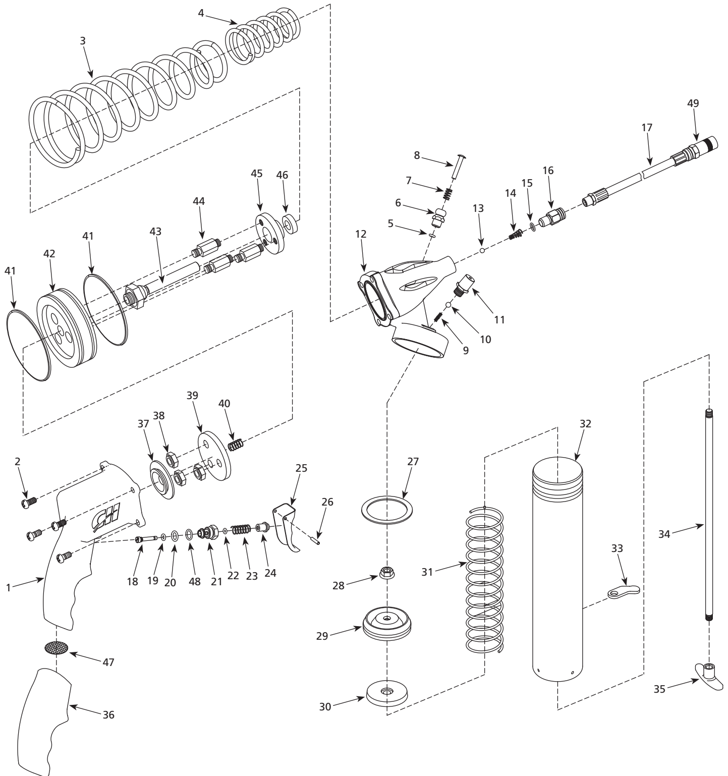
Figure 2 - Illustration de Pièces de Rechange
