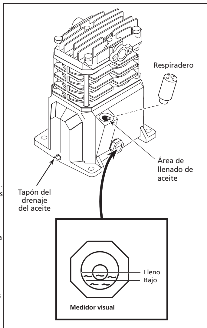
Figura 5 - Lubricacion
